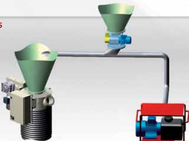
Butterfly valve with geared motor unit Drehklappe mit Motorantrieb Vanne papillon actionneur motorisé Compuerta de mariposa con mando motorizado Valvola a farfalla con comando motorizzato
